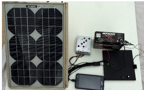
Figura 2. Circuito em funcionamento.
